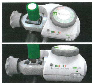
ダイヤル操作により操作性に特化したA案と、液晶表示により設定値を大きく表示したB案。両案とも意匠権を取得済。
