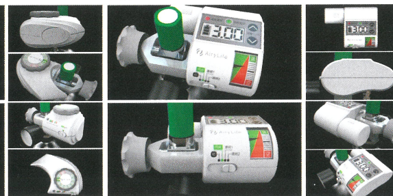
ダイヤル操作により操作性に特化したA案と、液晶表示により設定値を大きく表示したB案。両案とも意匠権を取得済。
