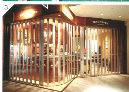
1／「イスターカーテン」用の金属レールをしなやかに曲げていく曲げ加工設備 2／曲げ加工設備を使い、金属レールが直線(左)から半径30センチの急カーブ(右)に変身する 3／都心の店舗に設置した曲線タイプの「イスターカーテン」。導入した曲げ加工設備を使えば、さらに小半径の曲線にも対応できる
