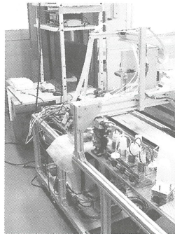
試作中の円筒形容器側面全周に直接印刷するプリンタ
