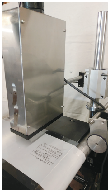
UVインクジェットプリンターPJ-600。印字幅は54ミリで二連すれば108ミリまで印字できる
