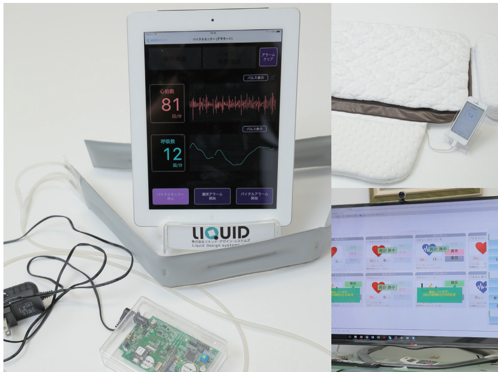
▲試作品「バイタルセンサー」と「表示用アプリケーション」(写真左)／枕部分のセンサーでバイタル信号をモニタリングしてスマホで表示(写真右上)／現在ではクラウドで複数名の情報を集中管理も可能(写真右下)
