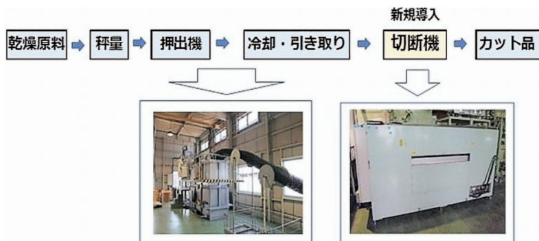
図1 PlaRain®の生産工程図
