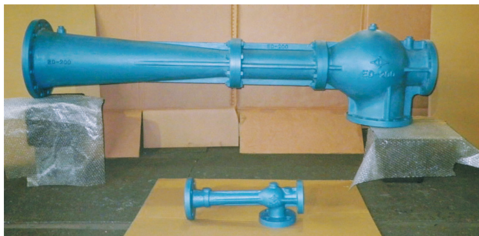
図1 製品となったエダクター (小さなものが当初開発品)
