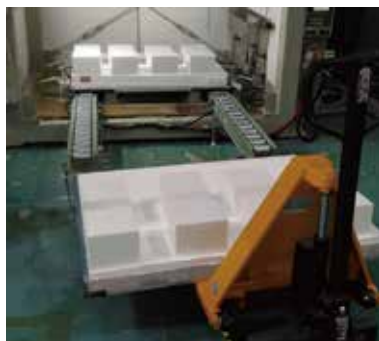
導入した段取り替え装置と3次元切削機
