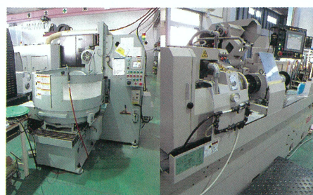
本事業後に導入したロータリー研削盤とCNC円筒研削盤
