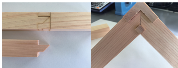
レーザー跡と切断後（左）、ホゾ穴の結合部分（右）
