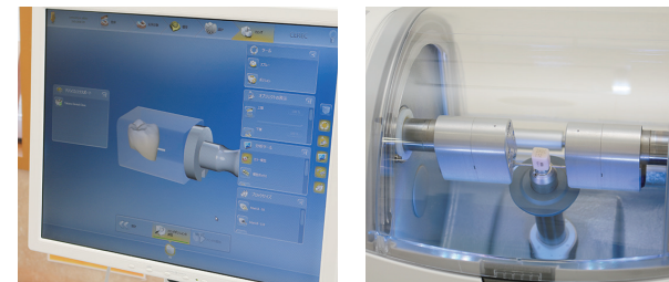
▲スキャンしたデータに基づいてモニター上でデザインし、そのデータを元に自動で削り出される
