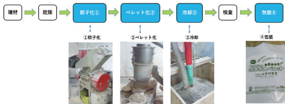
図2 ペレット製造設備と製造工程
