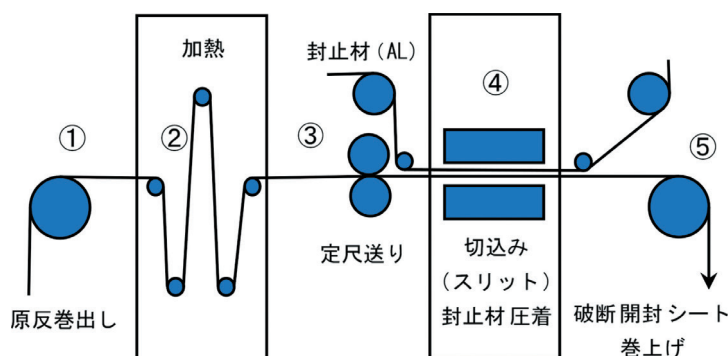
図2 破断開封シート加工工程
