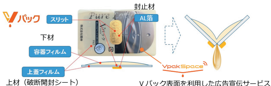
図4 Vパックのしくみ
