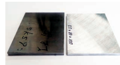
脱炭層(黒皮)除去前(左)と除去後(右)のゲージ鋼板
