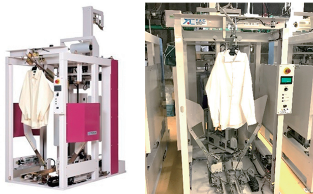
導入設備：Yシャツ自動立体包装機
