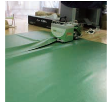
自走式溶着機
