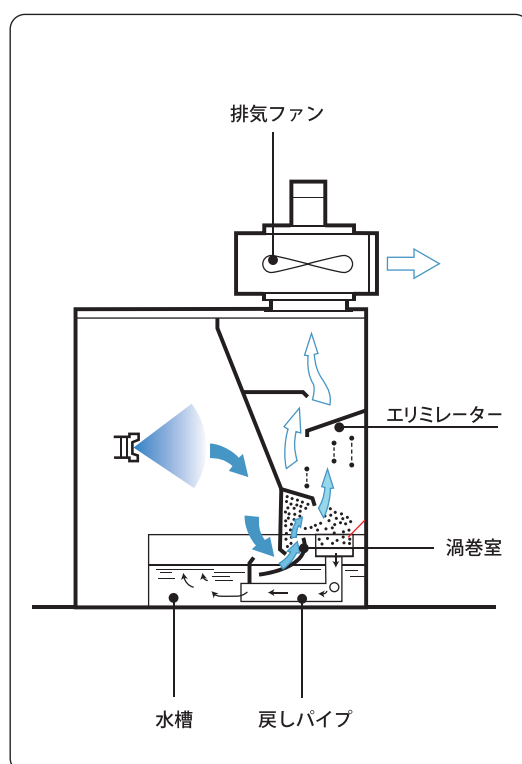
水洗式は塗料ミストが水に付着することを利用して捕集する。
