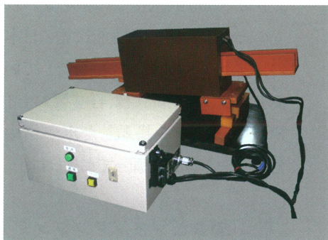
小型・シュータータイプ脱磁装置 ベアリング専用シューター式 PSD 型
