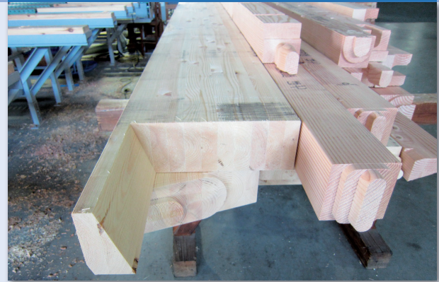
5軸加工機で加工した製品
