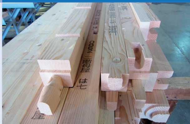
プレカット製品
