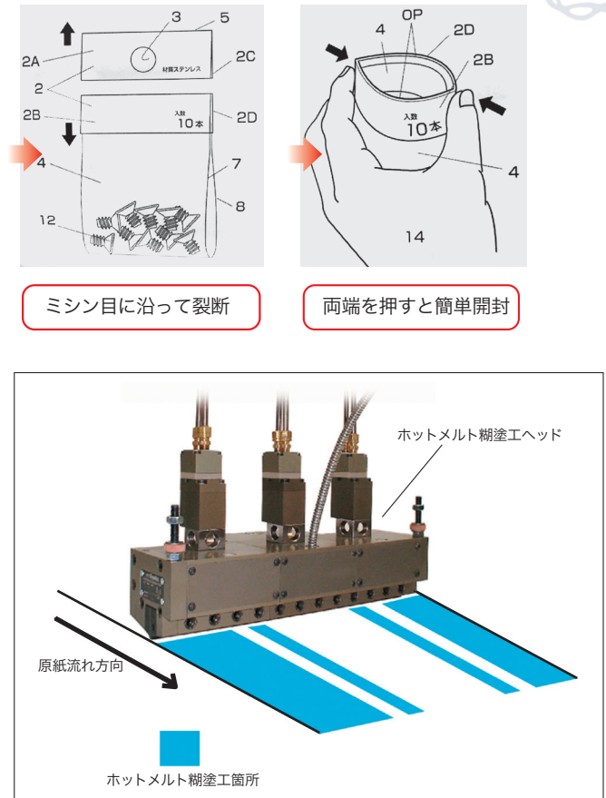
ホットメルト糊塗工イメージ
