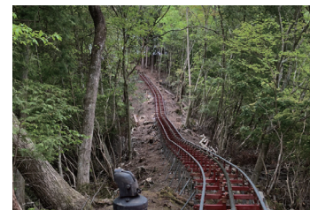
モノレール設置工事
