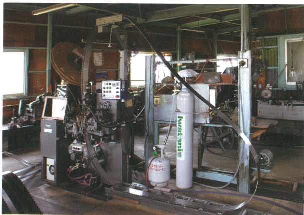
▲新たに導入したステライト・ハイス帯鋸自動溶着機
