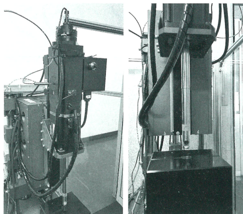
調整中の試作機とブロー部分
