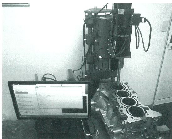
実証試験中の試作機
