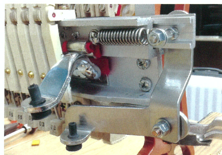
ベルクランク
