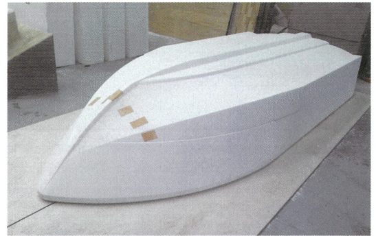
ボートのウレタンマスター型
