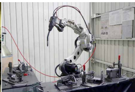
受託量増に伴い溶接ロボットを増設
