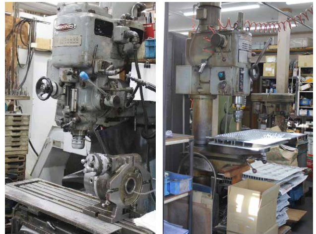
丁寧に使われてきた汎用工作機械
