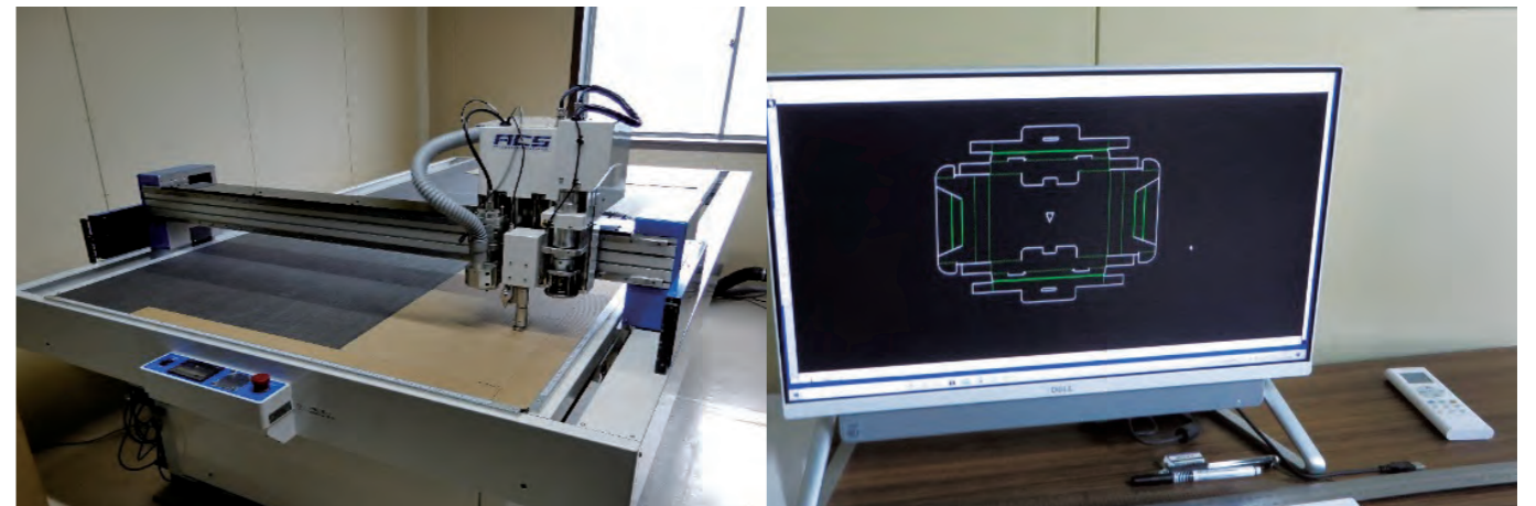
平成31年度ものづくり補助金事業(高度連携促進補助金事業)で導入されたレシプロカッター/CADシステム
