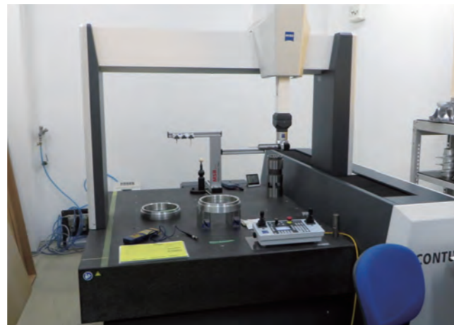
3次元測定器
